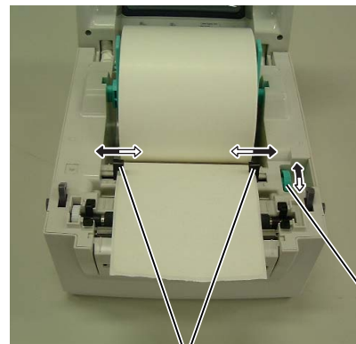
Guide carta
